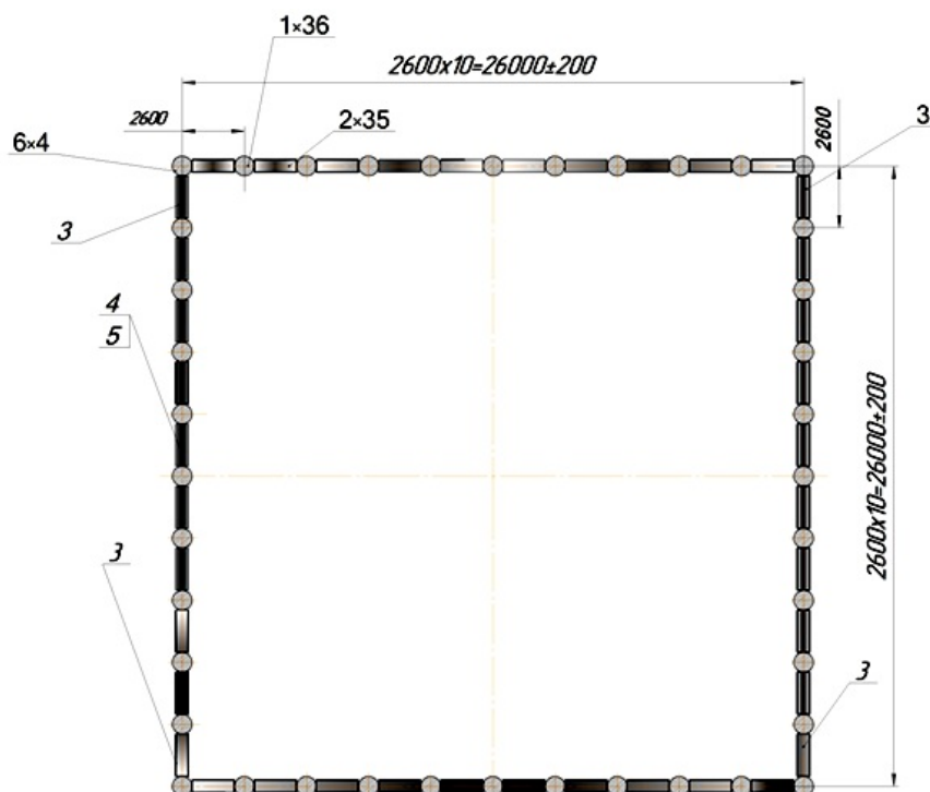
Рисунок 1.1- Ограда метеорологическая ОМП. Габаритный чертеж
